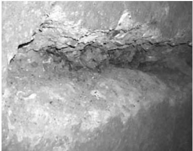
Očiščena razpoka v steni vodne celice
