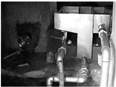
Vgrajevanje umirjevalnika vode v Zakojci
