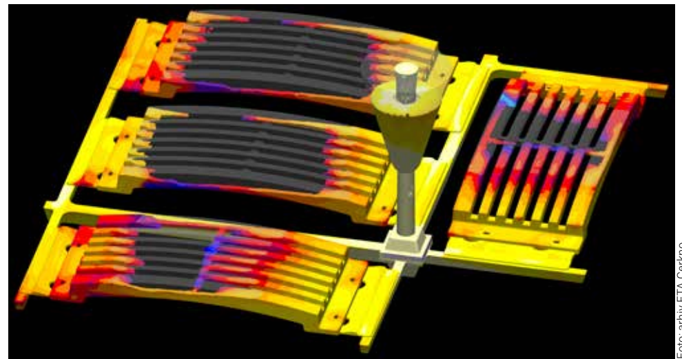
Simulacija ulivanja rešetke za zunanji del ohišja peči na lesne pelete.
